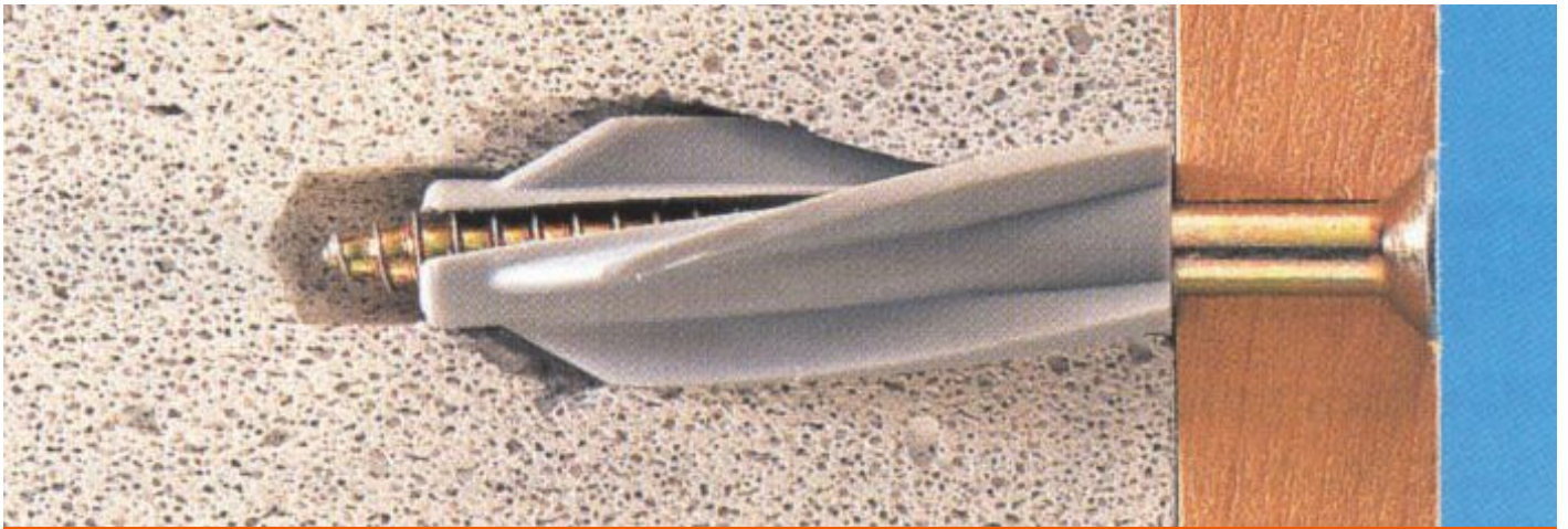
Fig. 28: Taquete Fischer para concreto celular AAC.
