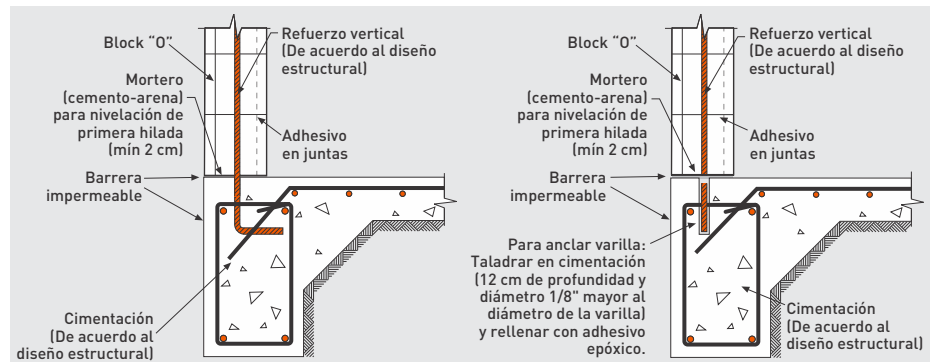
Fig. 7: Anclaje de refuerzo vertical en cimentación.
