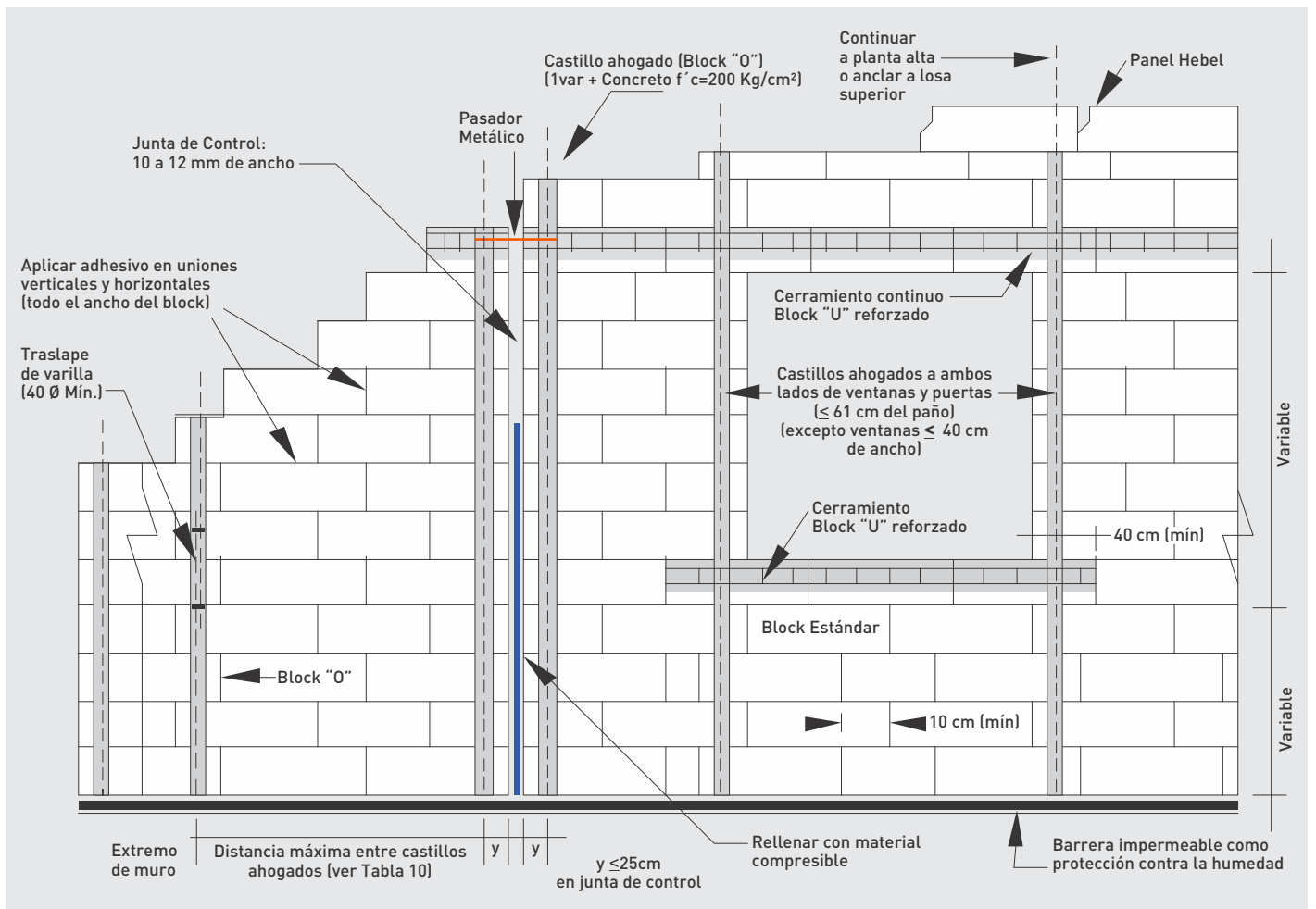
Fig. 20: Detalles constructivos para una correcta instalación del block Hebel.
